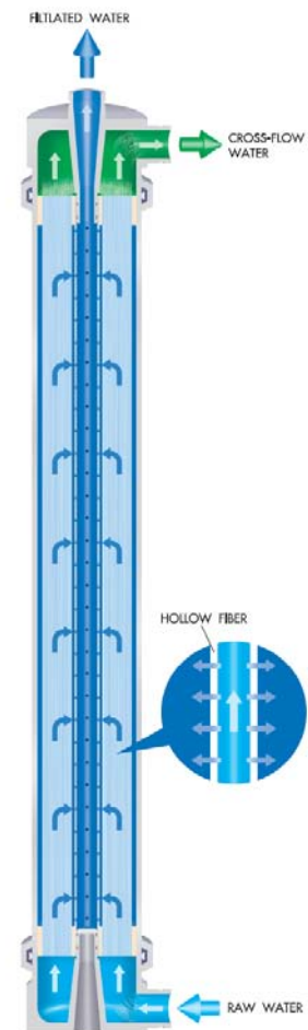
UF membrane module Model UPF0860
