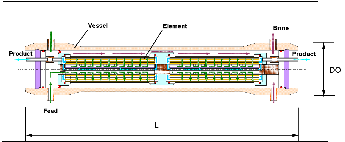
Module Dimension
